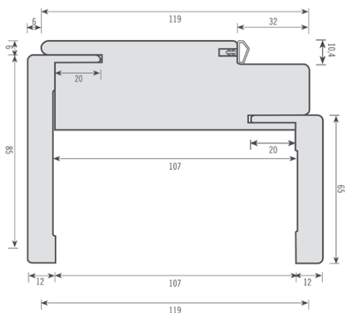
Particolare TELAIO
